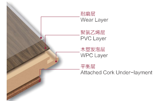
地板结构图 Structure
